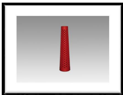
Proizvod Code : B 34A Dimenzije 36 * 63 * 280mm Materijal PP / Glass PP Težina 75gr.± 2gr.
