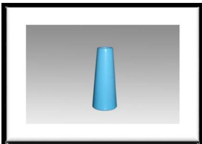
Proizvod Code : A 78X1 Dimenzije 28 * 59 * 170mm Material PP Težina 55gr.± 2gr.
