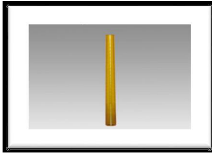
Proizvod Code : S 21A Dimenzije 16 * 22 * 260mm Material PC Težina 65gr.± 2gr.
