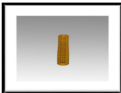
Proizvod Code :B 04CX1 Dimenzije 33 * 59 * 170mm Materijal Glass pp Težina 110gr.± 2gr.
